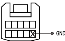
(空调面板后10PIN连接器端子示意图)
