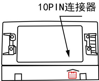
(空调面板后10PIN连接器位置示意图)
