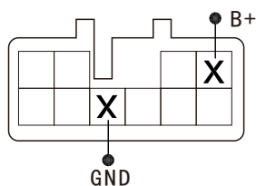
(10PIN连接器端子示意图)
