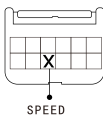
(12PIN连接器端子示意图)
